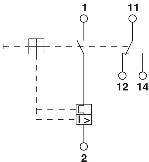
Kopplingsschema
