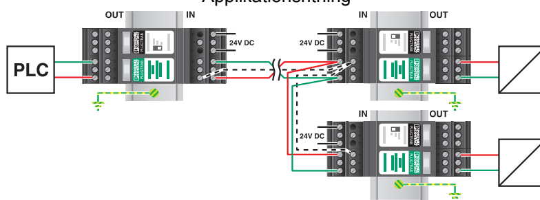
Applikationsritning
