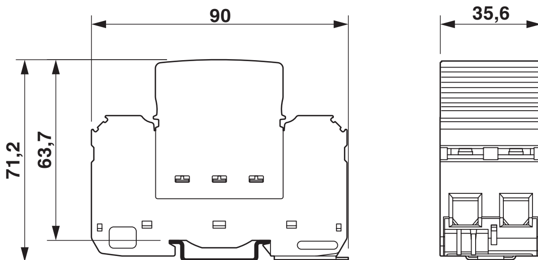
Måttskiss
