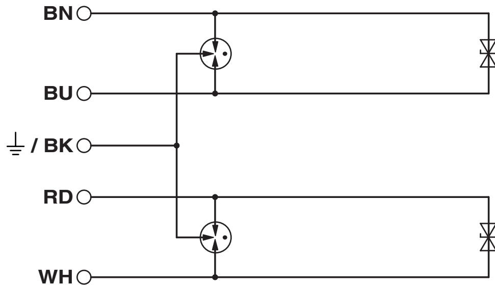
Kopplingsschema
