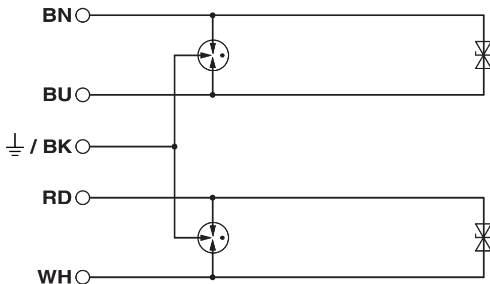
Kopplingsschema
