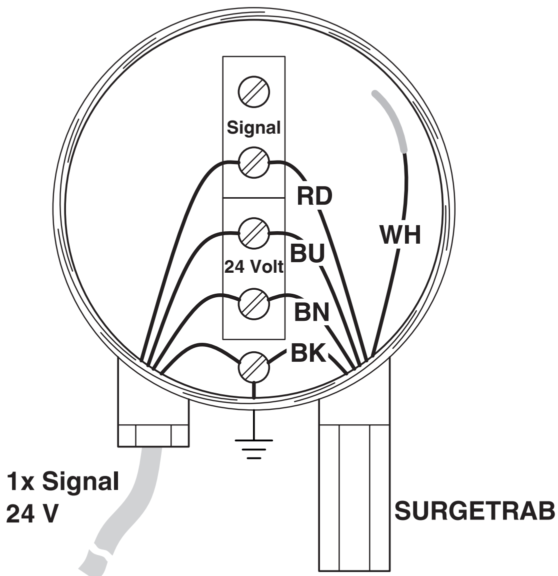
Applikationsritning
