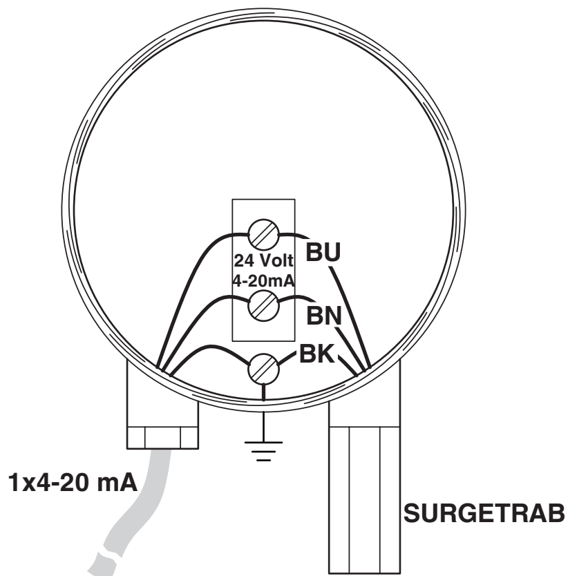
Applikationsritning
