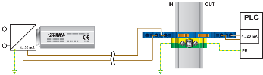
Applikationsritning
