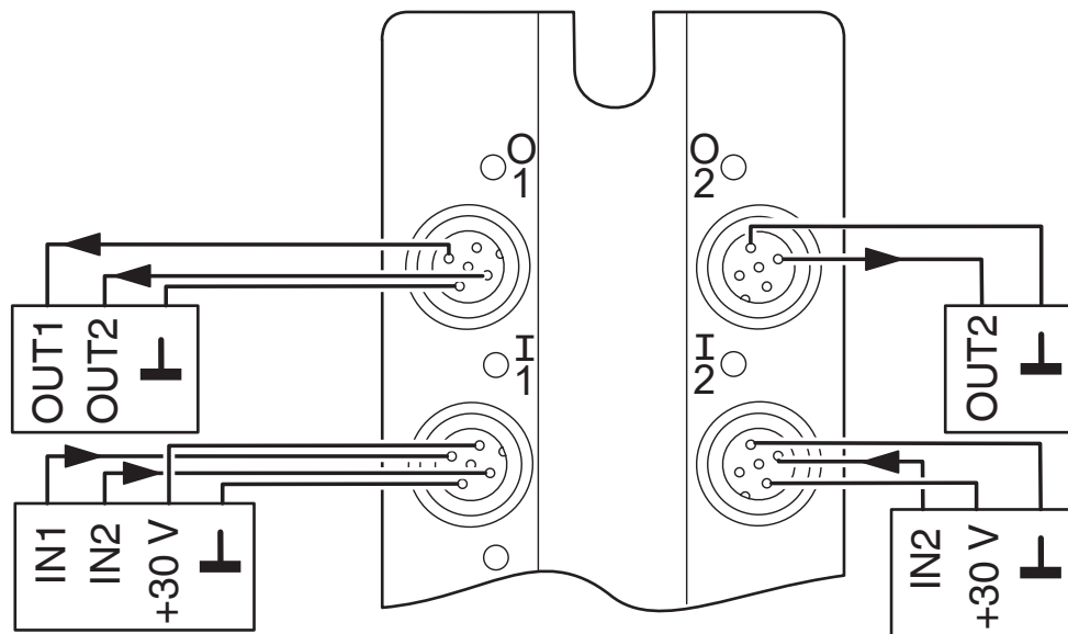
Anslutningsritning
