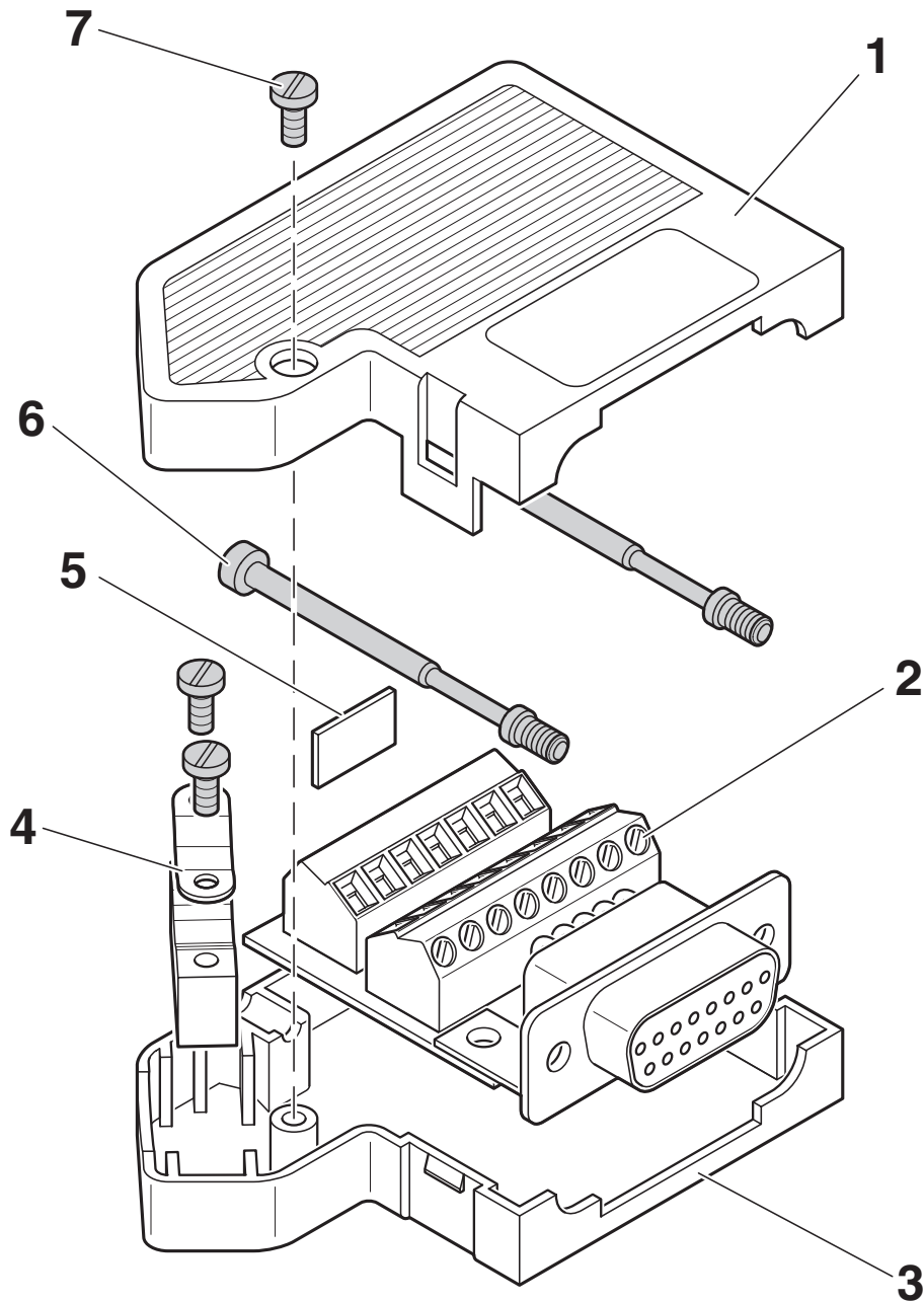
Schematisk ritning
