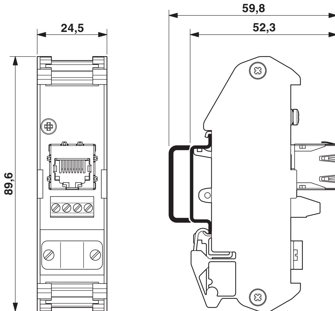
Måttskiss
