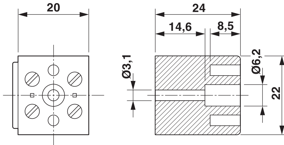
Måttskiss
