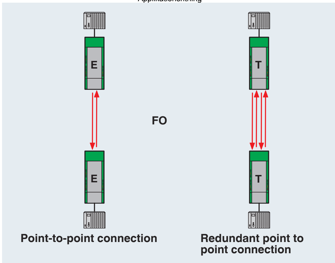
Redundant punkt-till-punkt-anslutning
