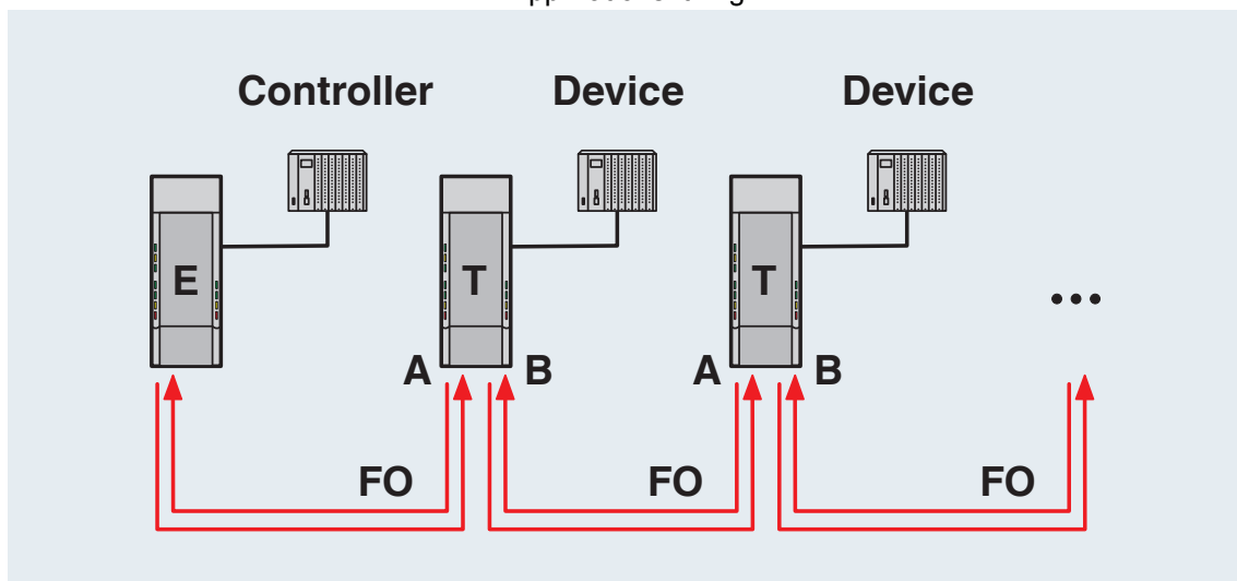
Controller-Device-linjestruktur
