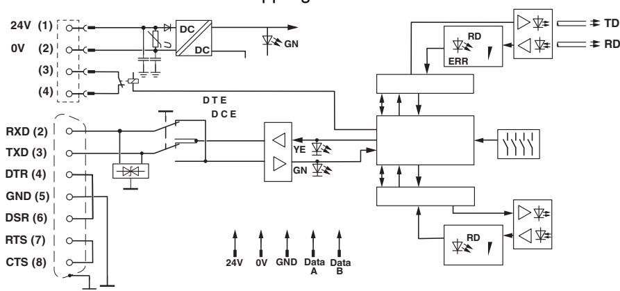
Kopplingsschema
