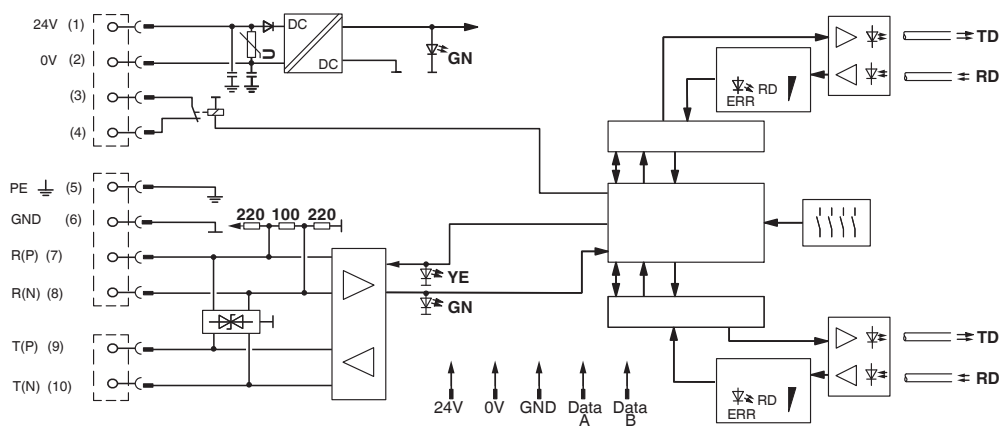
Kopplingsschema
