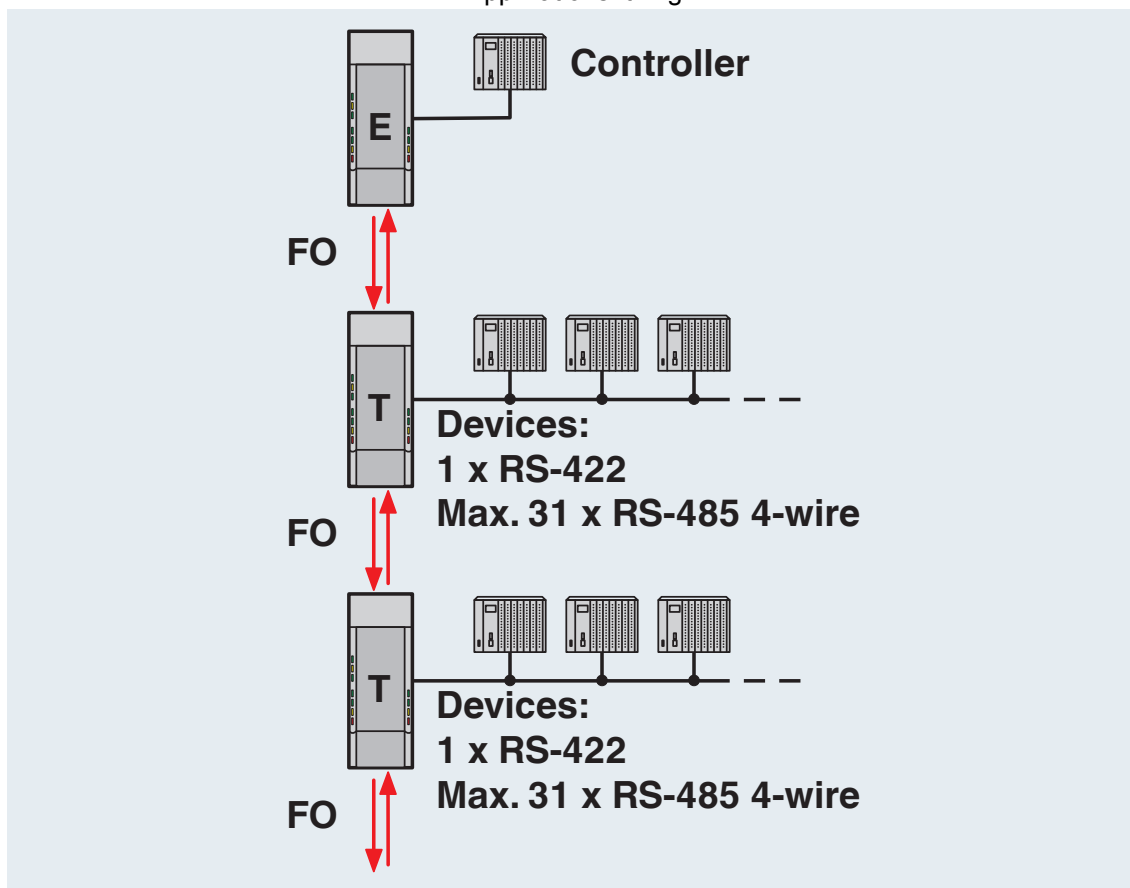
Controller-Device-linjestruktur
