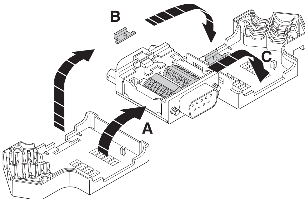
Schematisk ritning
