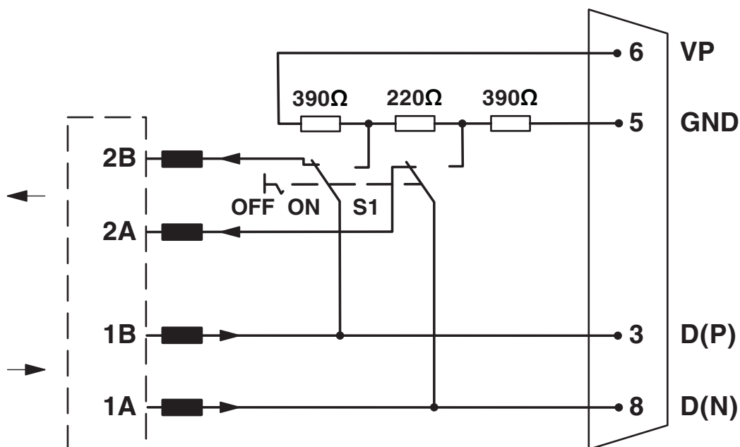
Kopplingsschema för kontaktserien SUBCON-PLUS-PROFIB/...
