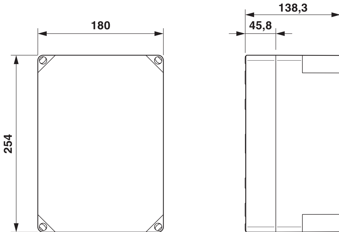
Måttskiss
