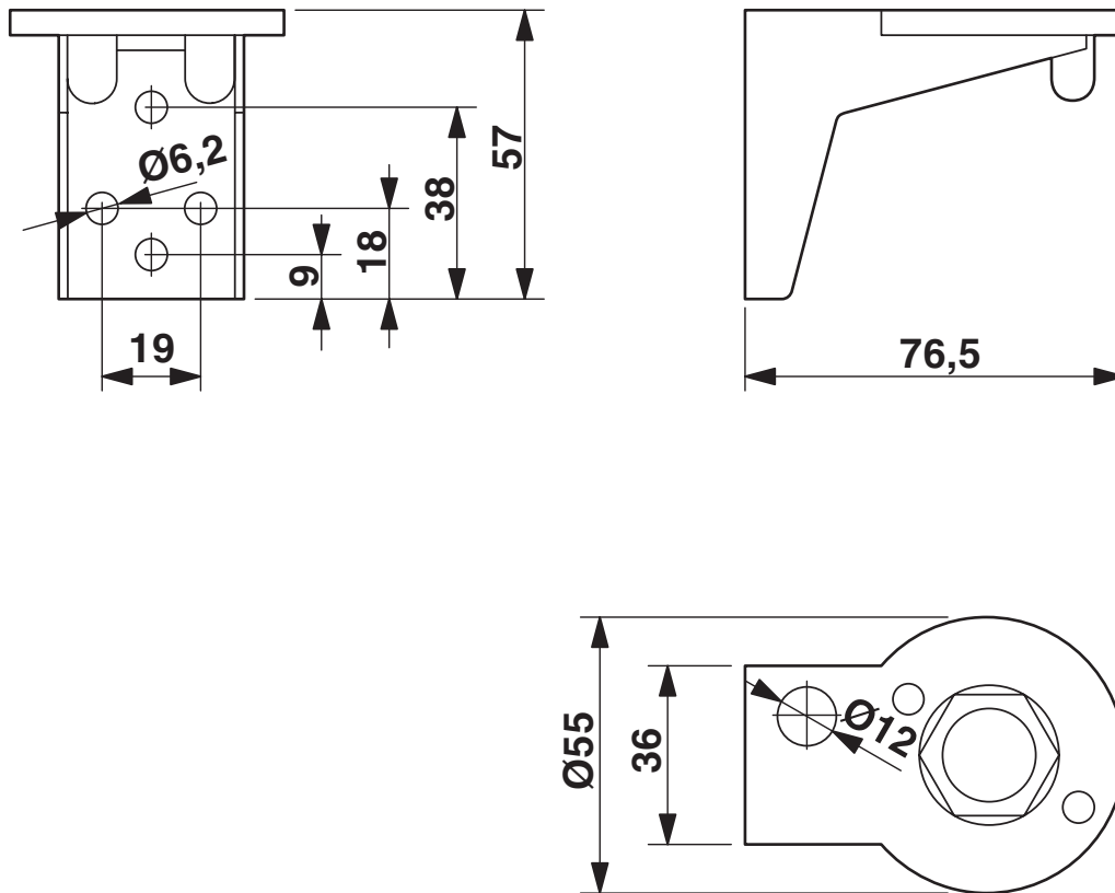
Måttskiss
