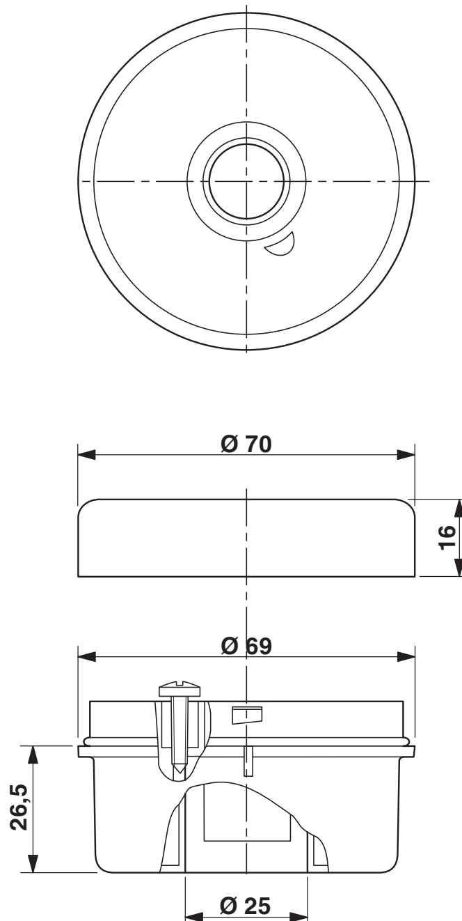
Måttskiss
