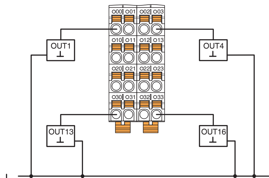
Anslutningsritning
