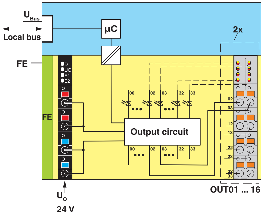
Kopplingsschema
