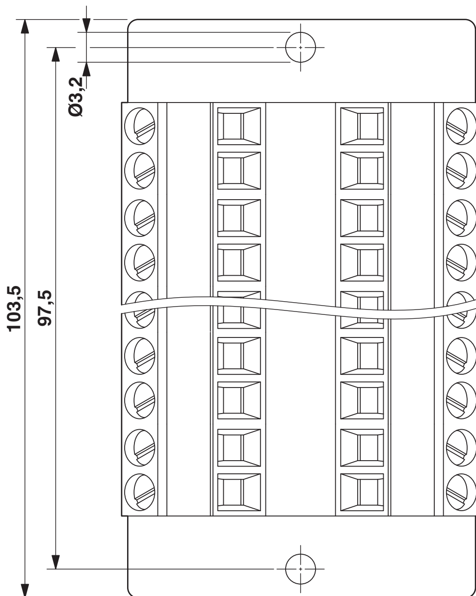
Måttskiss
