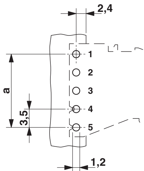
Borrplan/lödöns geometri
