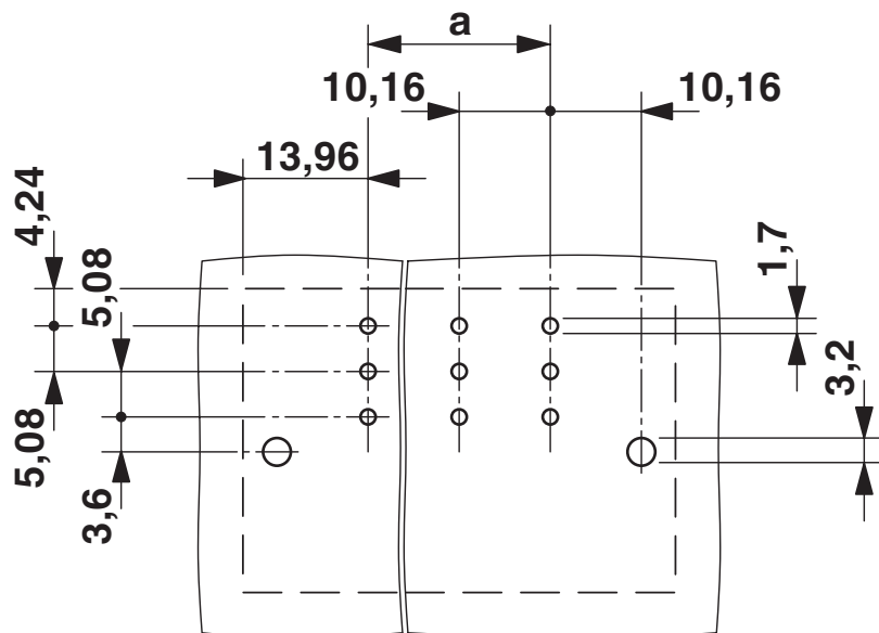
Borrplan/lödöns geometri
