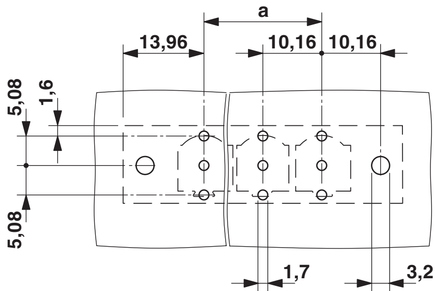
Borrplan/lödöns geometri
