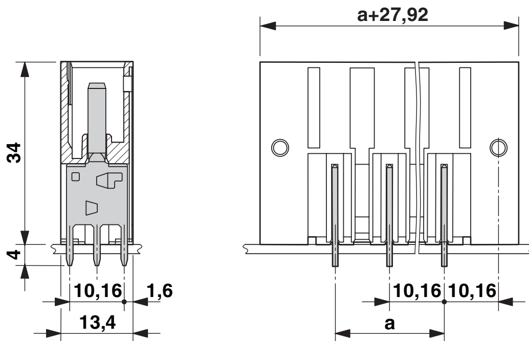
Måttskiss
