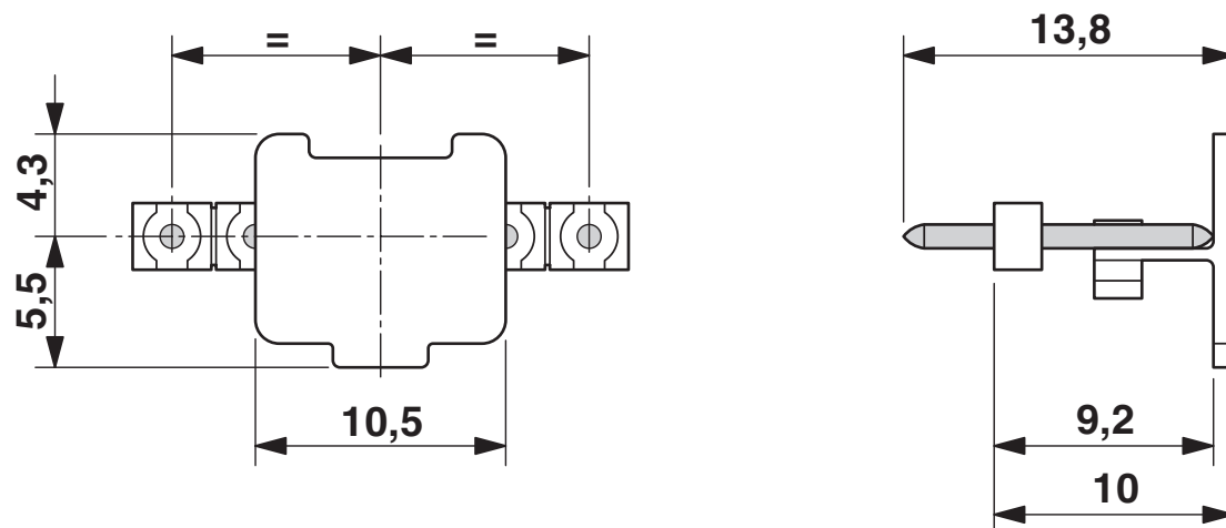
Måttskiss
