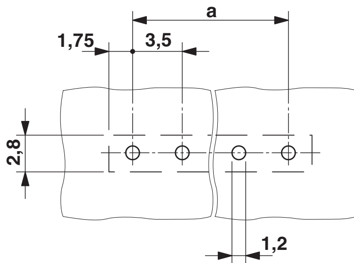
Borrplan/lödöns geometri
