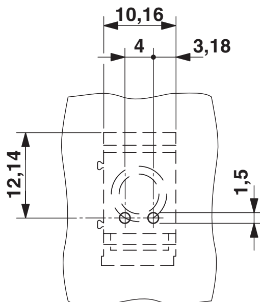
Borrplan/lödöns geometri
