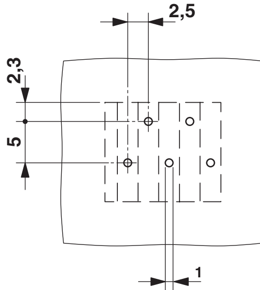
Borrplan/lödöns geometri
