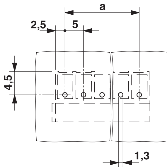
Borrplan/lödöns geometri
