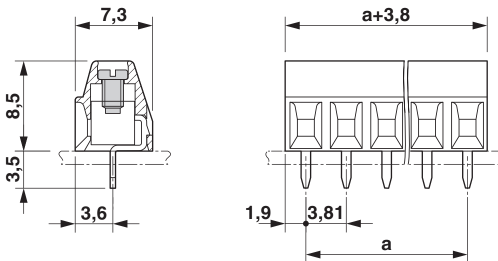
Måttskiss
