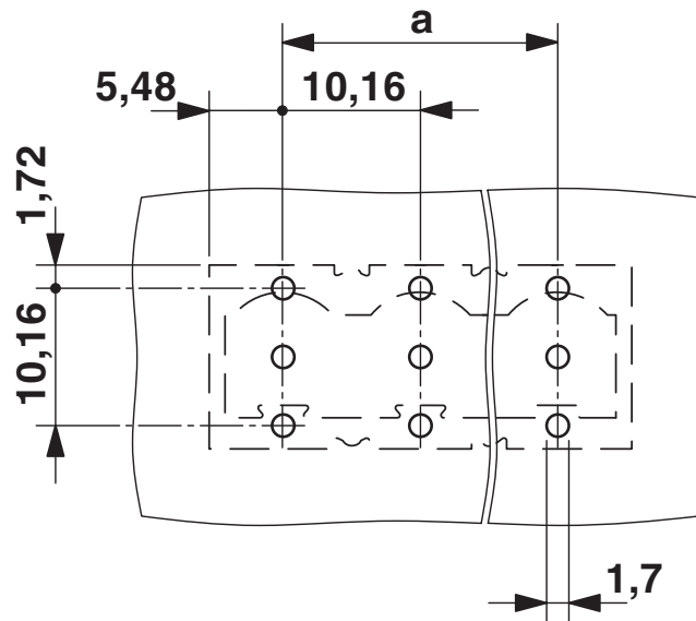
Borrplan/lödöns geometri
