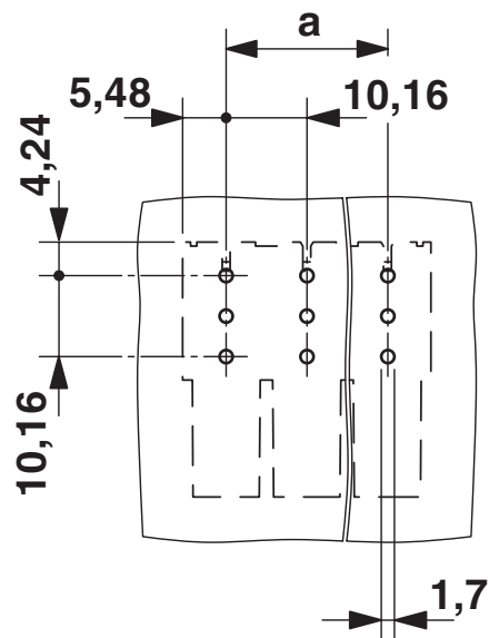
Borrplan/lödöns geometri
