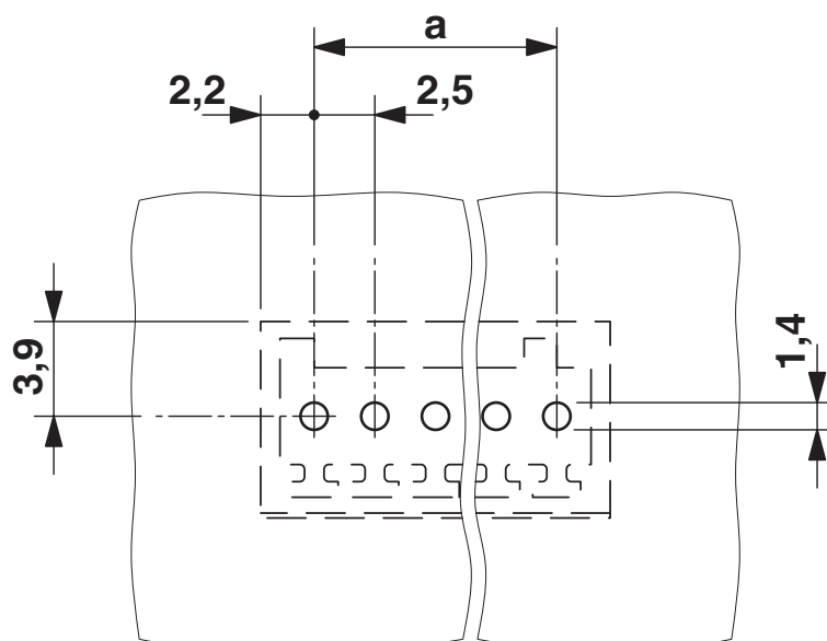
Borrplan/lödöns geometri
