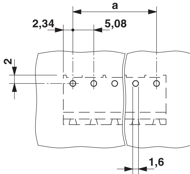
Borrplan/lödöns geometri
