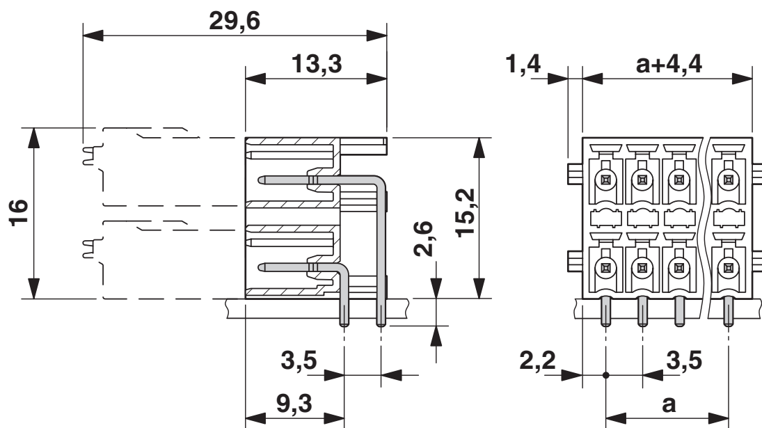
Måttskiss
