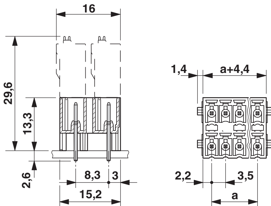
Måttskiss
