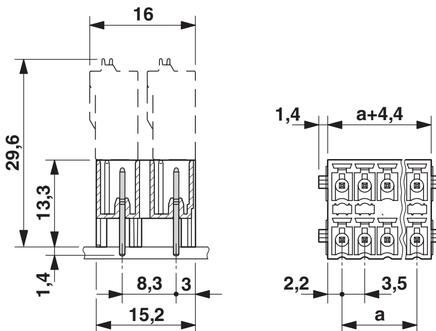
Måttskiss
