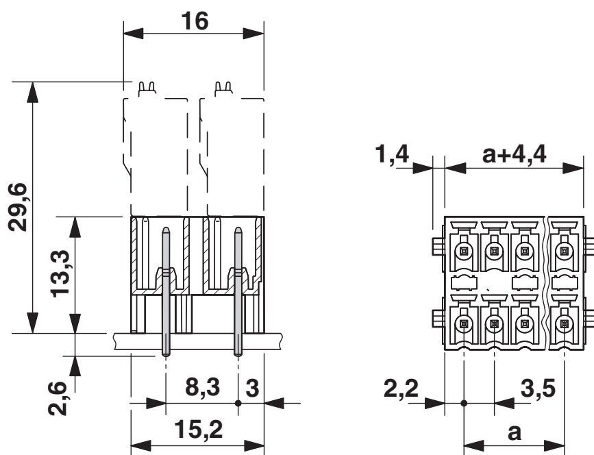
Måttskiss
