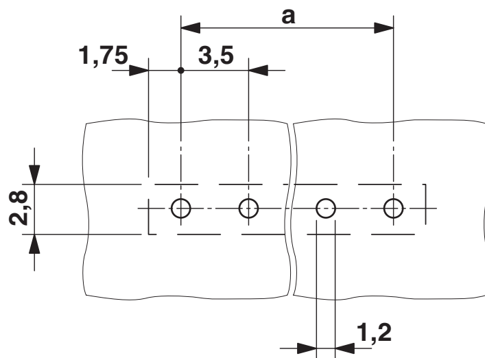
Borrplan/lödöns geometri
