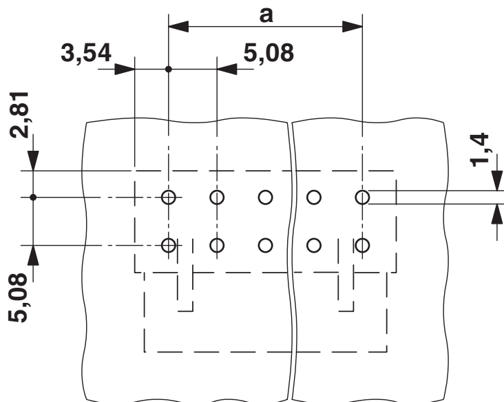
Borrplan/lödöns geometri
