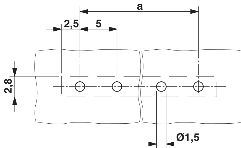
Borrplan/lödöns geometri
