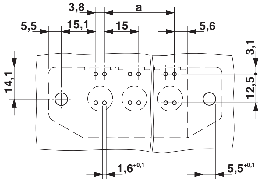
Borrplan/lödöns geometri
