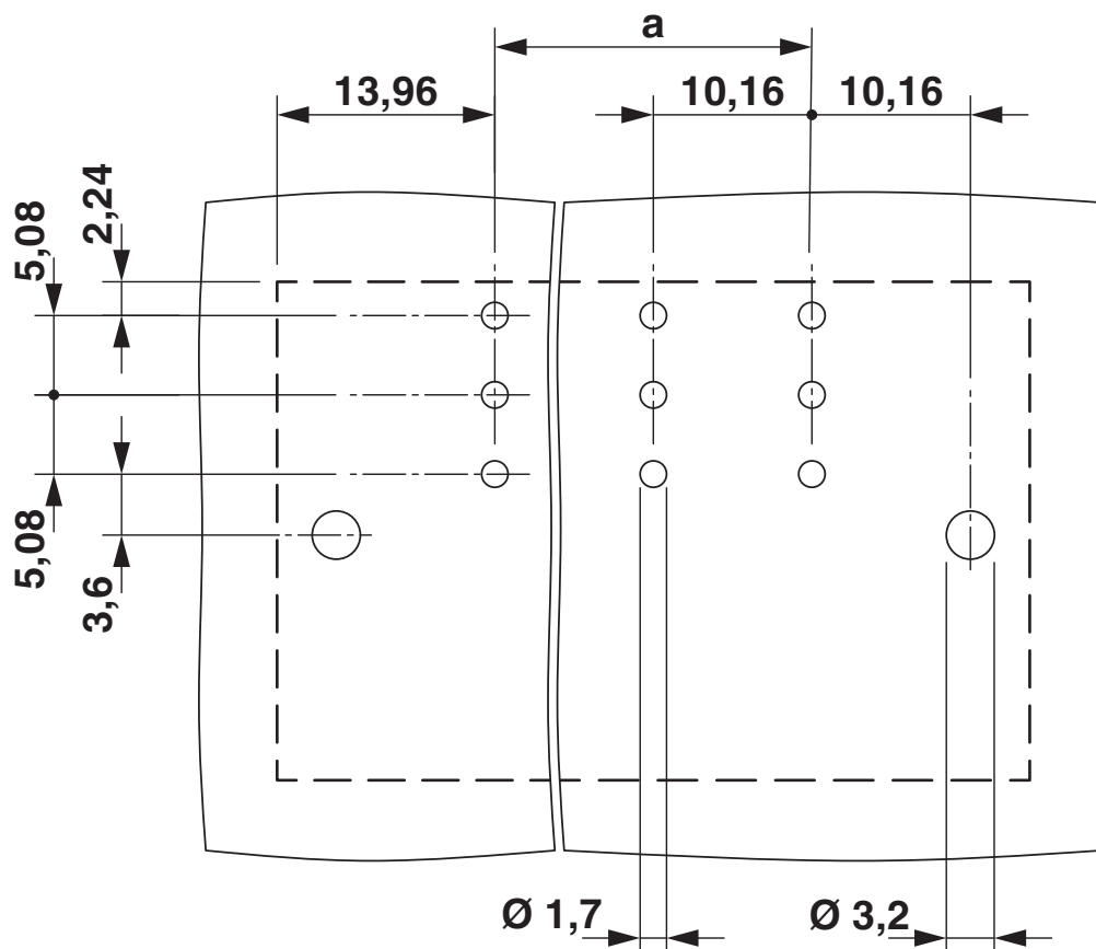
Borrplan/lödöns geometri
