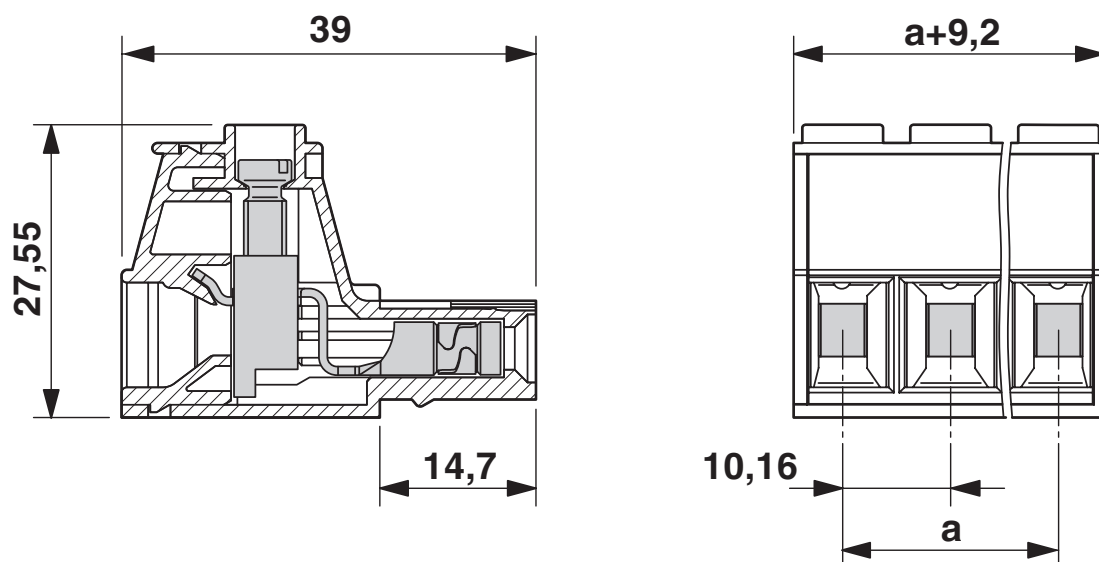
Måttskiss
