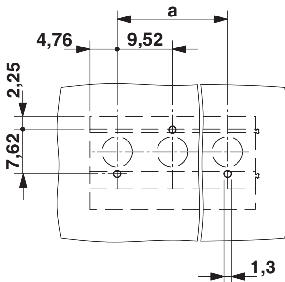
Borrplan/lödöns geometri
