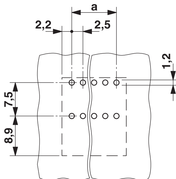
Borrplan/lödöns geometri
