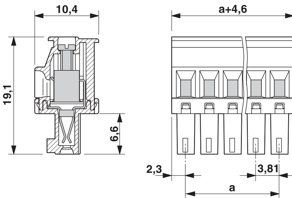
Måttskiss
