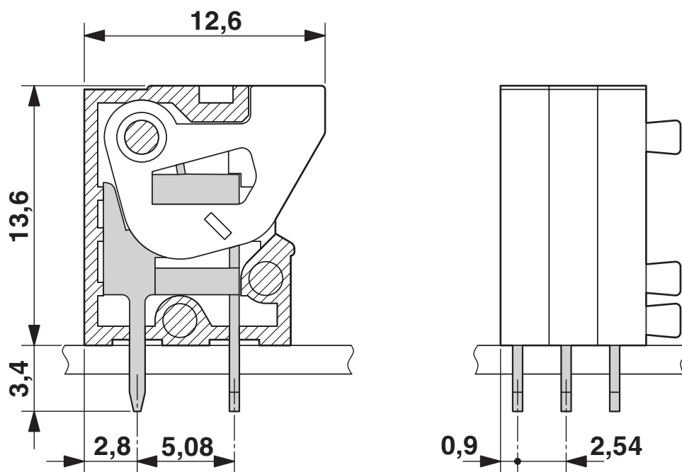
Måttskiss
