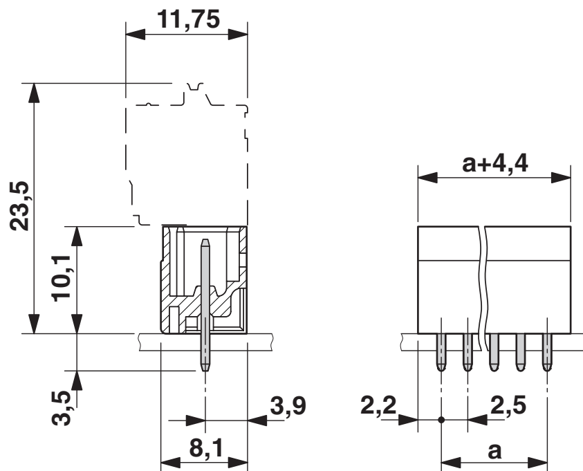
Måttskiss
