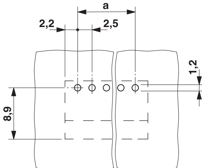
Borrplan/lödöns geometri
