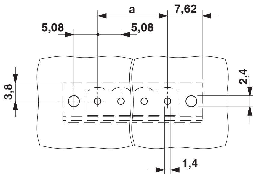
Borrplan/lödöns geometri
