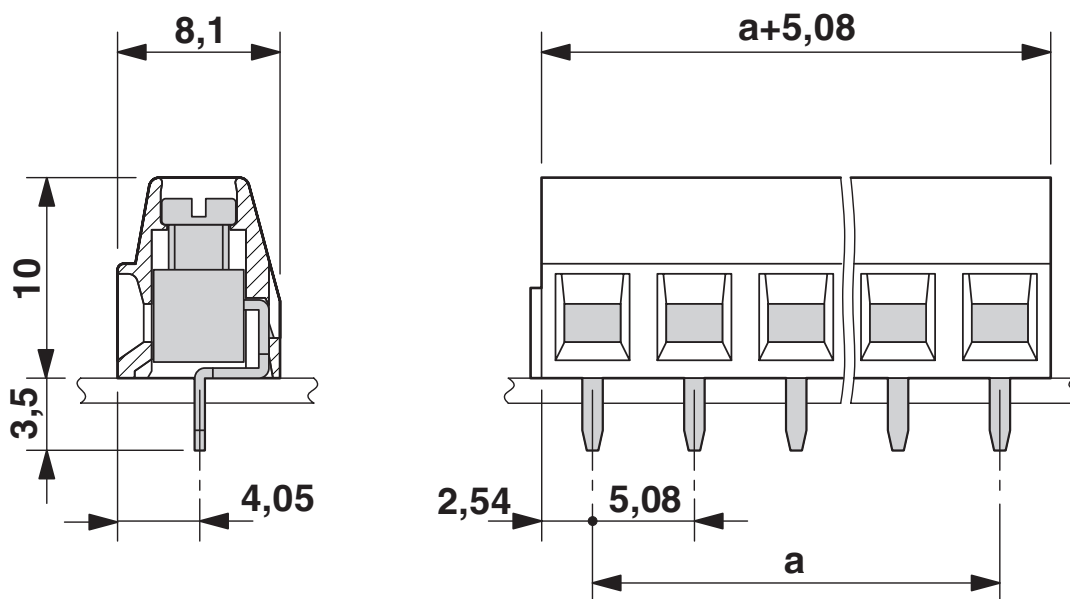
Måttskiss
