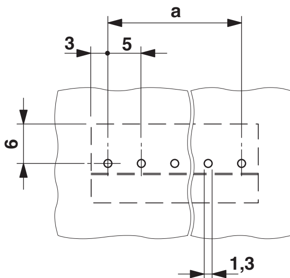
Borrplan/lödöns geometri
